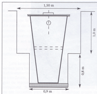
Tanque séptico en plástico reforzado con fibra de vidrio
