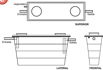
Tanque séptico en plástico reforzado con fibra de vidrio
