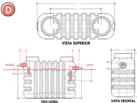
Tanque séptico en polietileno
