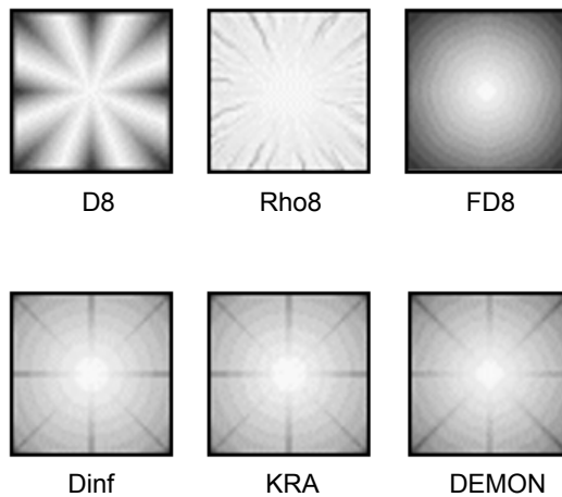
Figura 15.18: Representación del área acumulada sobre un cono circular según los principales algoritmos de asignación de direcciones de flujo (adaptado de [243])
