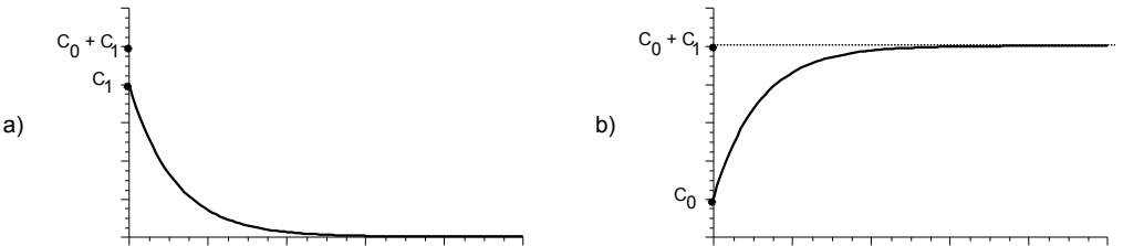
Figura 12.11: Relación entre correlograma (a) y variograma (b)
