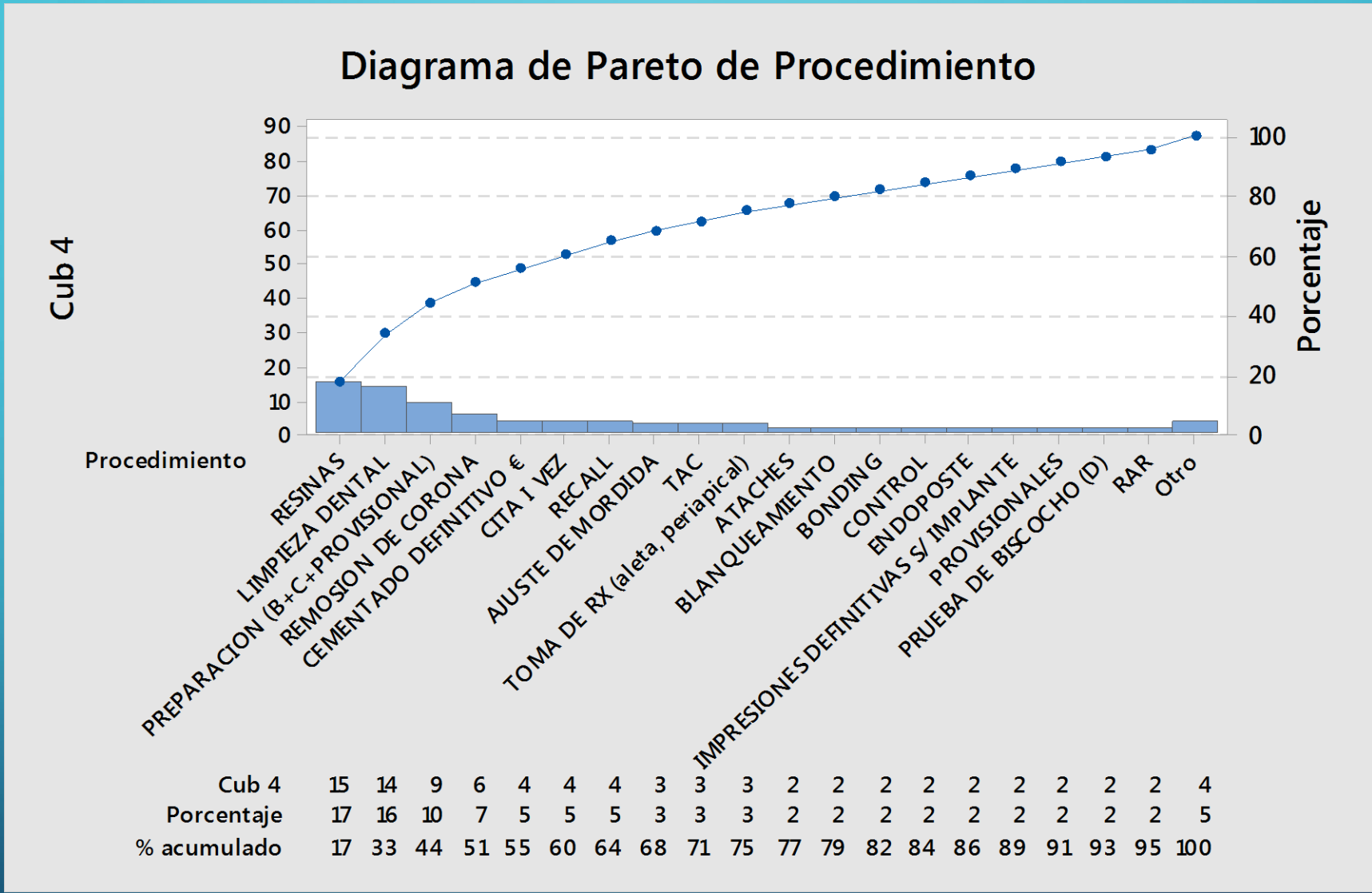
Figura 12. Diagrama de Pareto representado por el cubículo 4.
